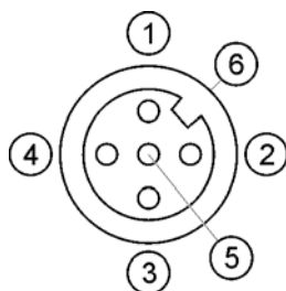
Разположение на щифтовете на буксата (в терминала)
