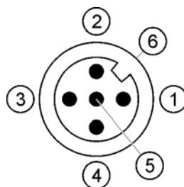
Разположение на щифтовете на щекера
