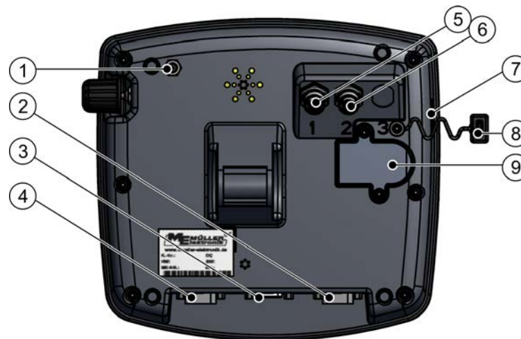
Задна страна на терминала. Вариант с GSM модем и изводи за камера
